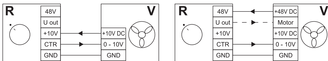
Schéma zapojenia ovládača
