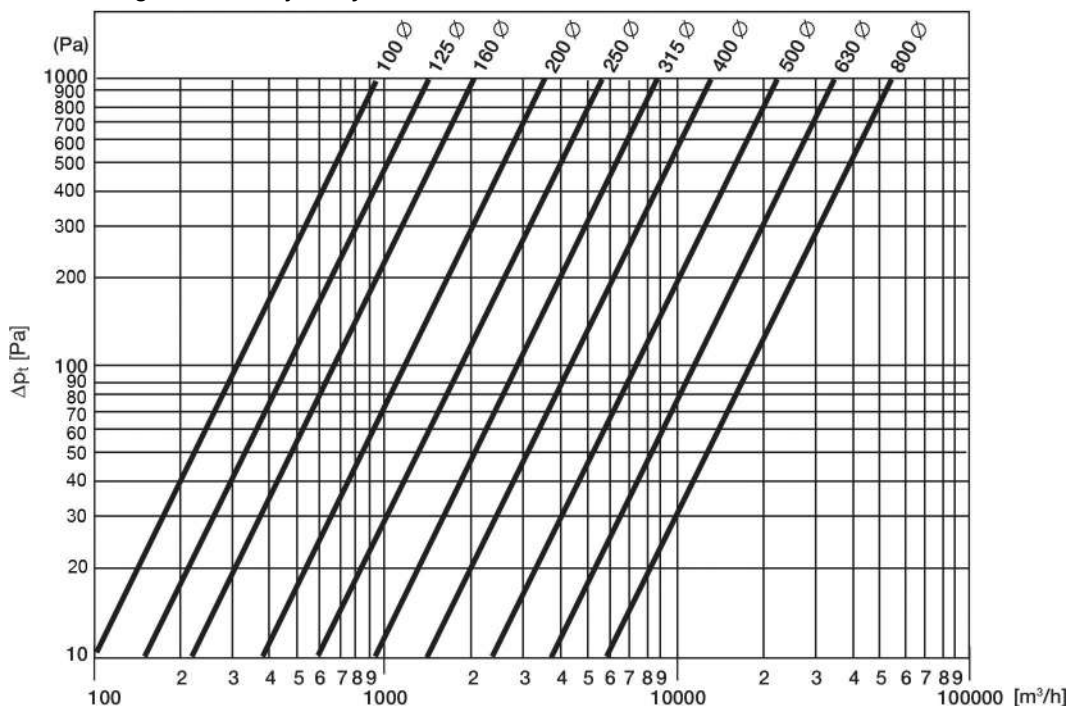
Diagram tlakovej straty
